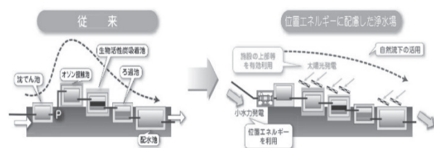
図3-32 エネルギー効率に配慮した浄水場の施設配 置（イメージ）
