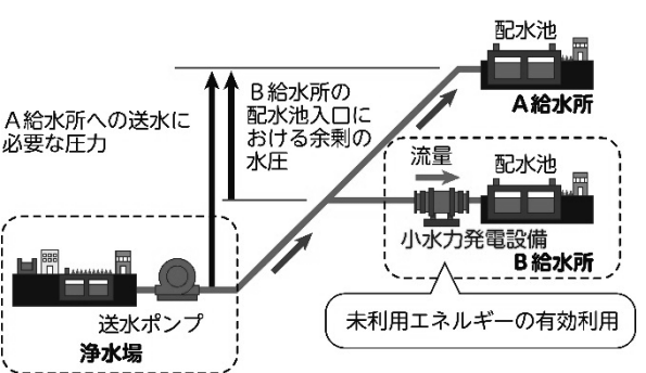
図3-30 余剰圧力を利用した水力発電イメージ
