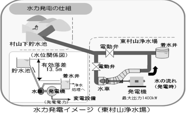
図3-29 高低差を利用した水力発電イメージ
