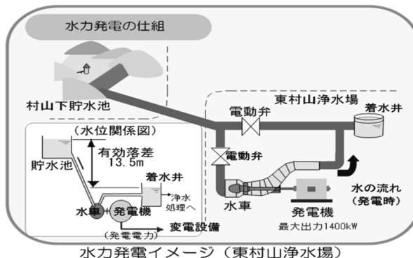
図3-28 高低差を利用した水力発電イメージ
