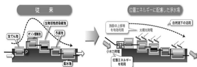
図3-31 エネルギー効率に配慮した浄水場の施設配置（イメージ）
