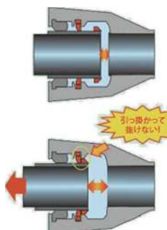
耐震継手管の構造(イメージ図)
