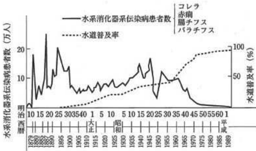
水道普及率と水系伝染病患者数の推移 (出典 改訂 水道のあらし 日本水道協会)
