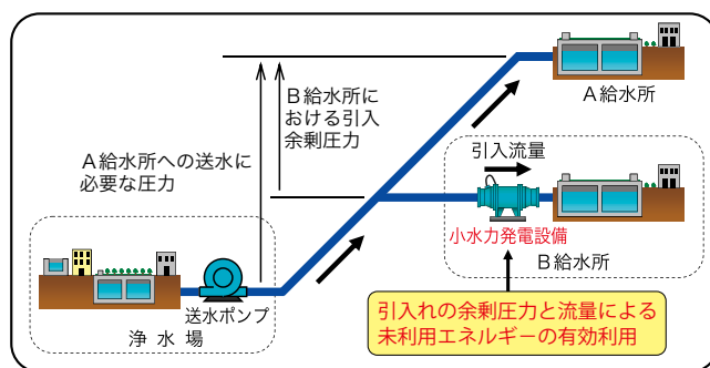
給水所における小水力発電設備
