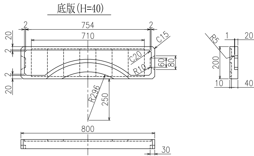
底版断面詳細図
