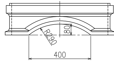
調整リング (H=50)
