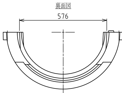
裏面図
