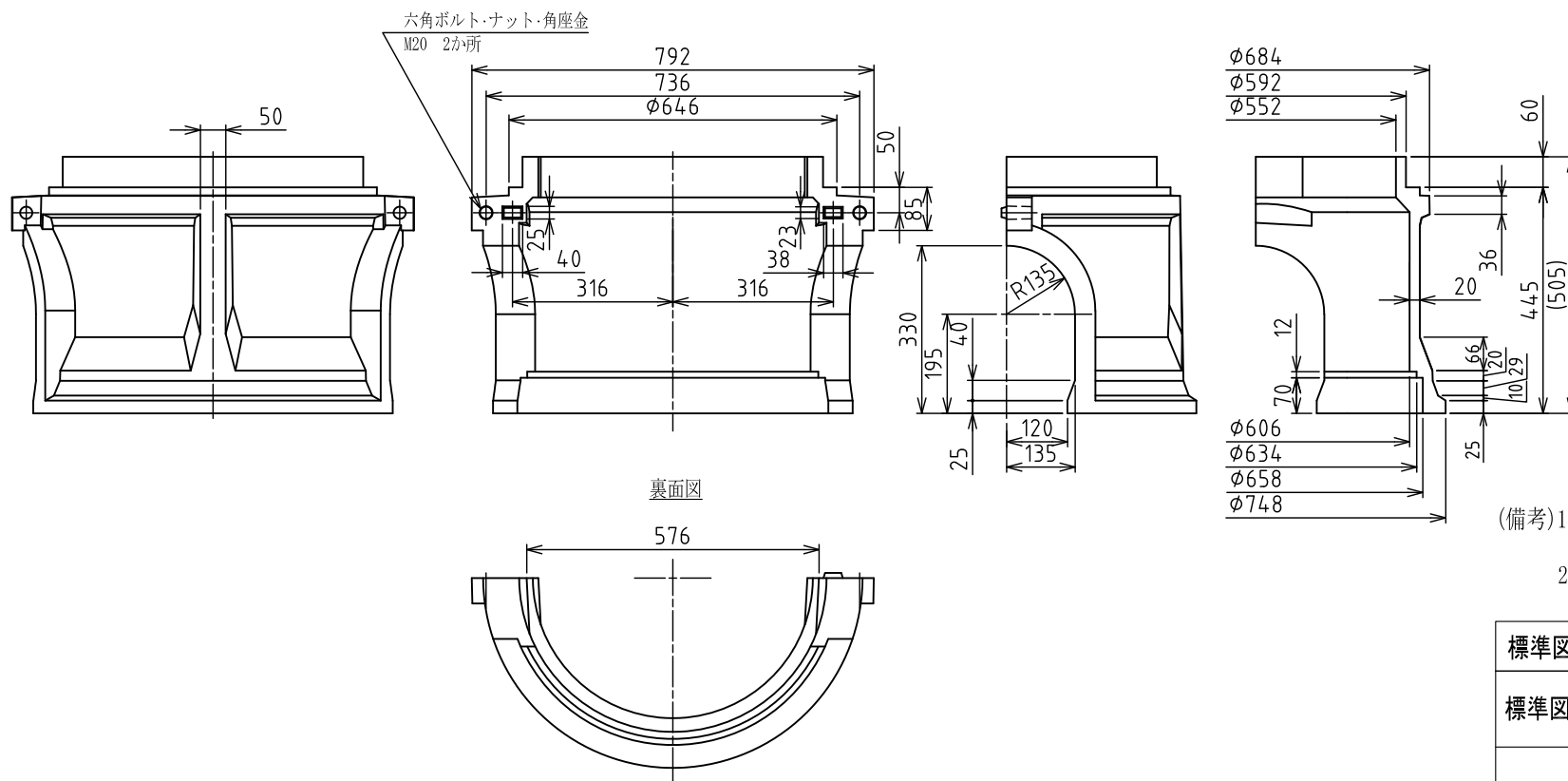
正面図
