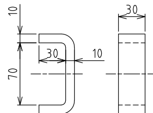
連結金具詳細図
