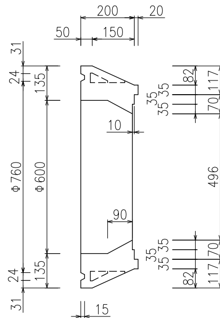
② - ② 断面図
