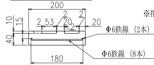
円形消火栓用レジンコンクリート製ボックス材料表
