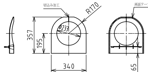
側面図
