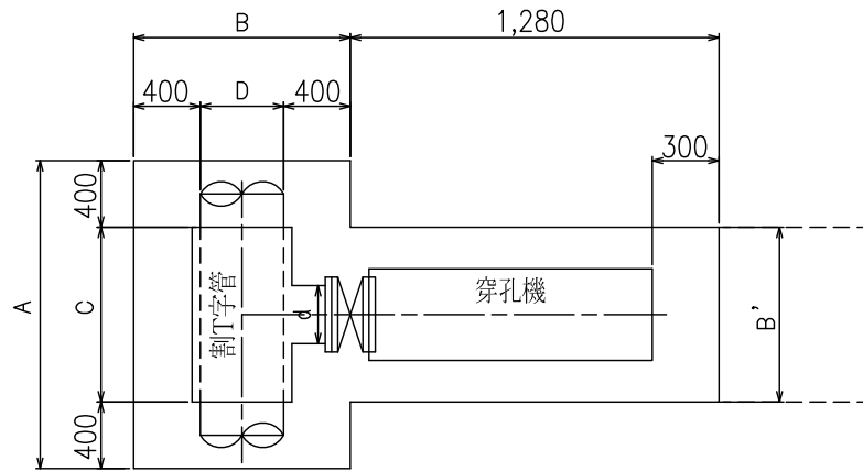
掘削平面図
