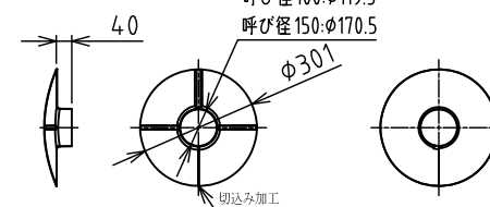
側面図
