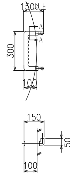
足掛金物W300
