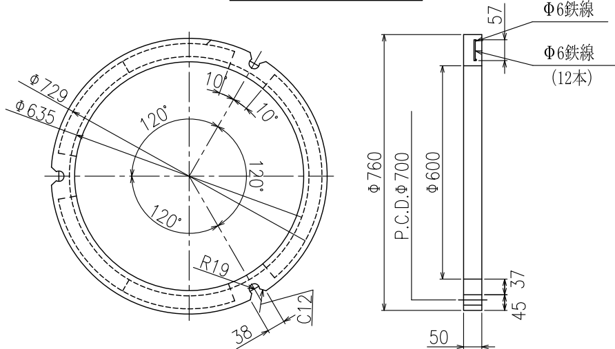
調整リング (H=50)
