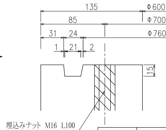
詳細図
