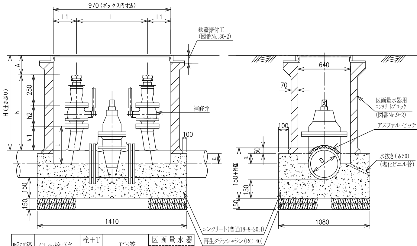
補修弁 2種
