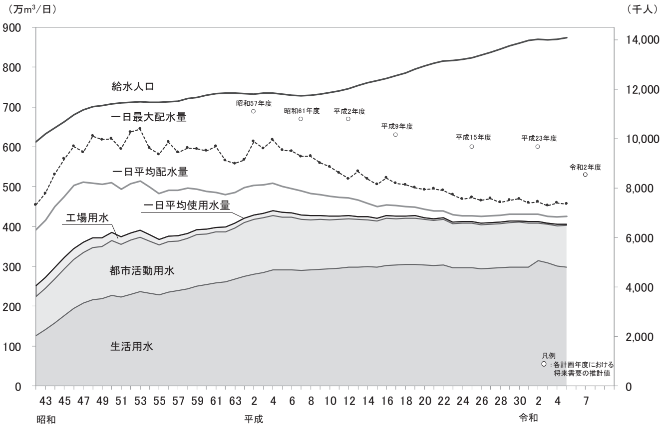
図2-1 一日最大配水量、一日平均配水量、一日平均使用水量（生活用水、都市活動用水、工場用水）及び給水人口（区部及び29市町 （注1） ）
