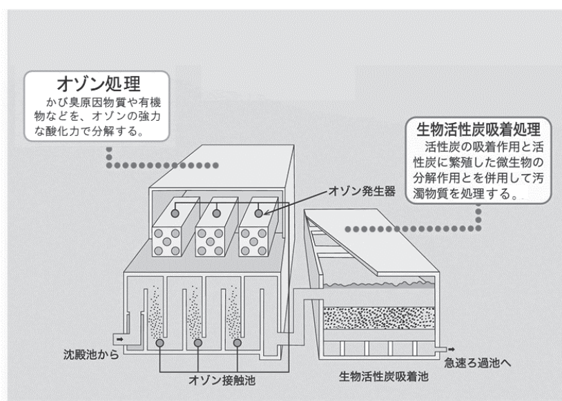
図２－９ 高度浄水処理の仕組み（金町浄水場）
