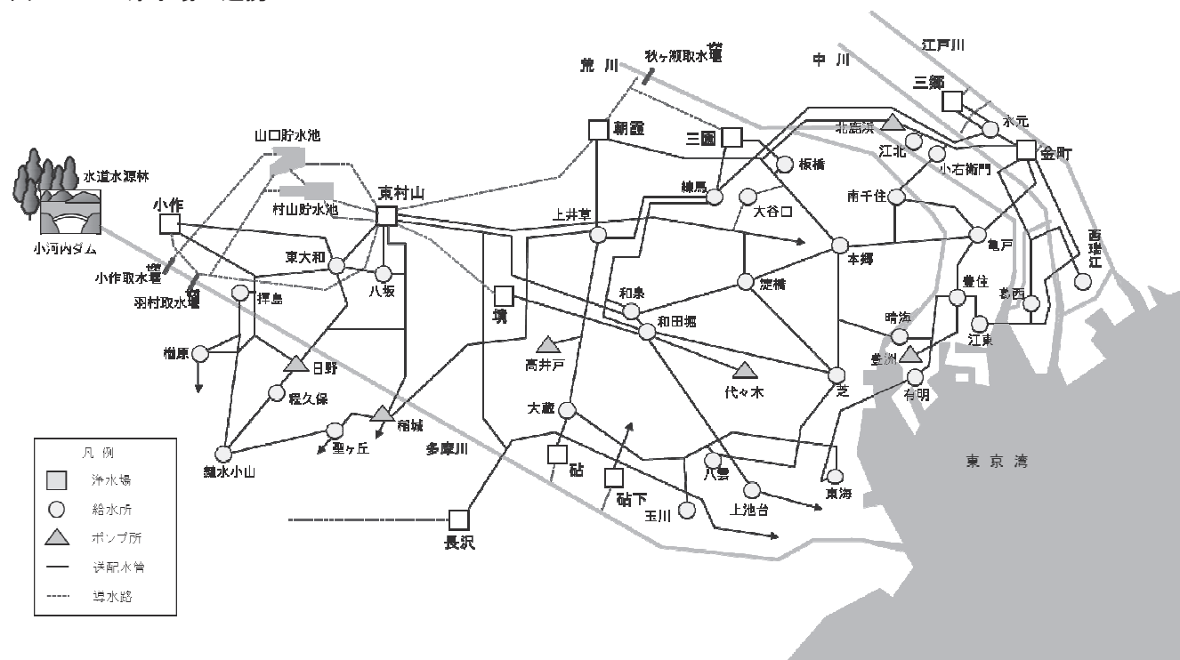
図 2-11 浄水場の連携
