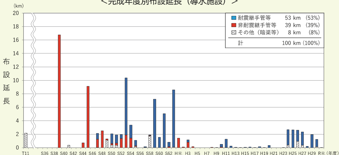
&lt;完成年度別布設延長（導水施設）&gt;
