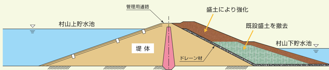
<村山上貯水池堤体強化の概略断面図>
