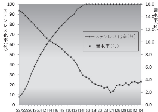
図3-23 ダクタイル化率と配水管自然漏水修理件数の推移（左図）及び給水管のステンレス化率と漏水率（右図）
