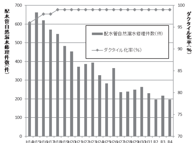
図3-23 ダクタイル化率と配水管自然漏水修理件数の推移（左図）及び給水管のステンレス化率と漏水率（右図）
