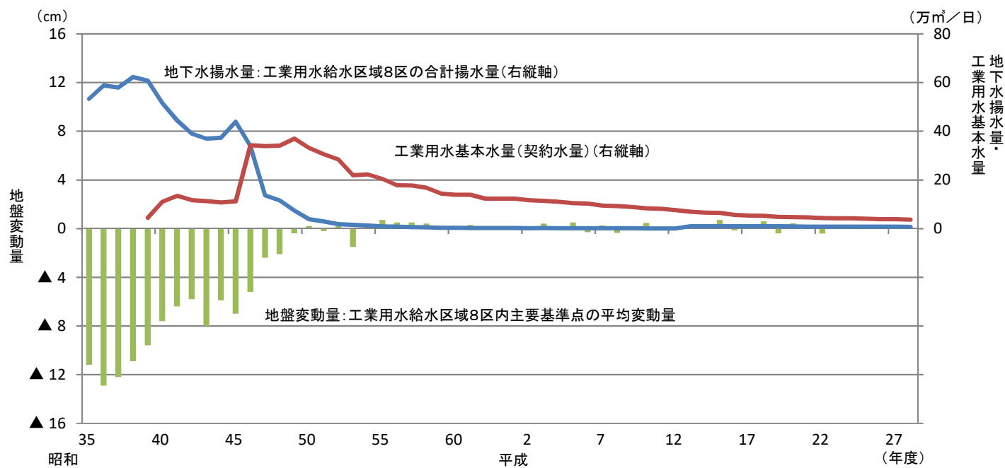
「地下水揚水量と地盤変動量の推移」
