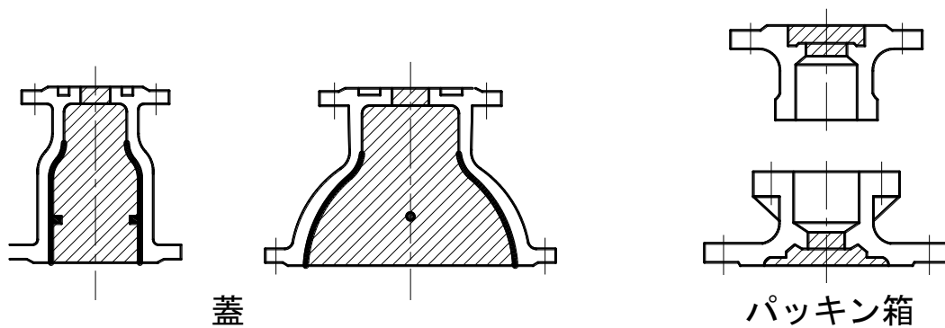
図－１．３ 蓋及びパッキン箱の内面塗装範囲及び塗装検査の範囲
