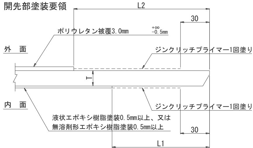
塗覆装要領図（１）
