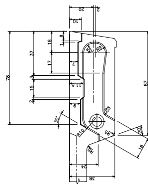
鐵蓋蝶番部詳細圖
