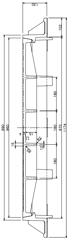
A-A断面図
