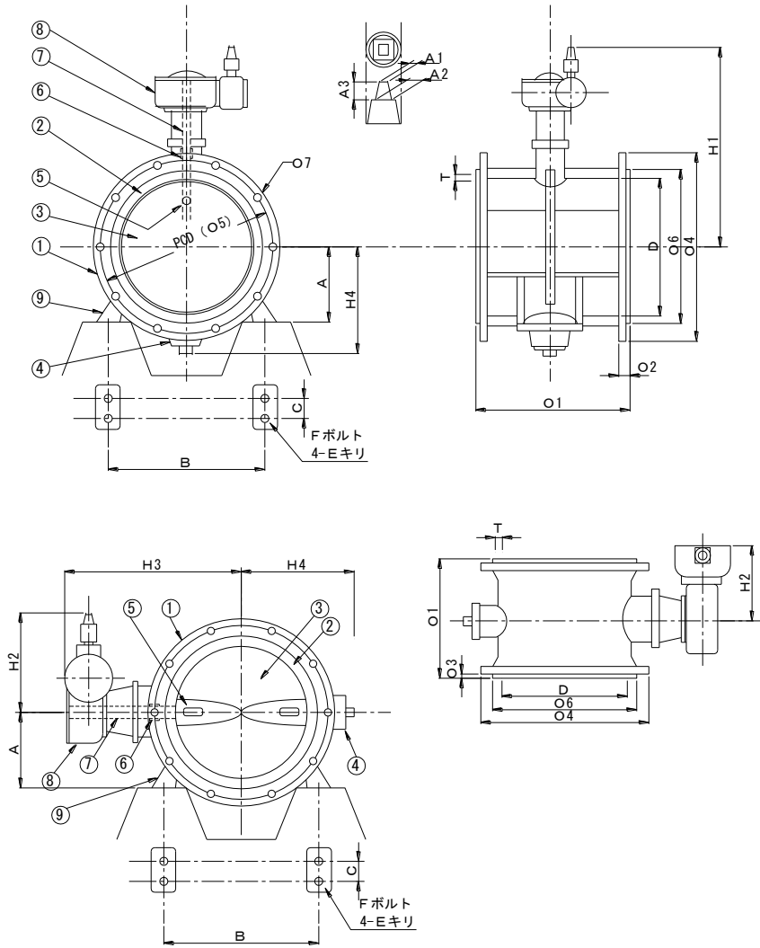
付図－１ 水道用ダクティル鑄鉄製バタフライ弁の構造・形状
