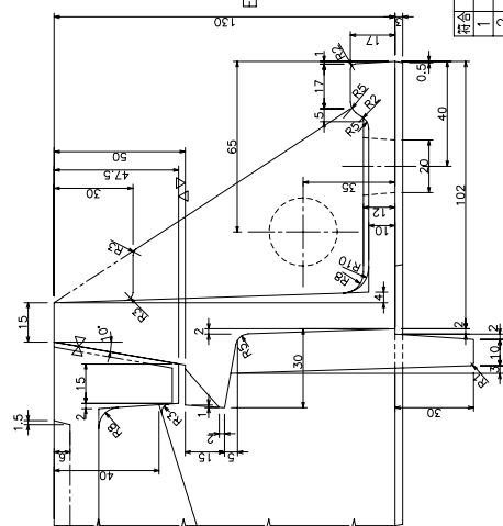
C-C断面图
