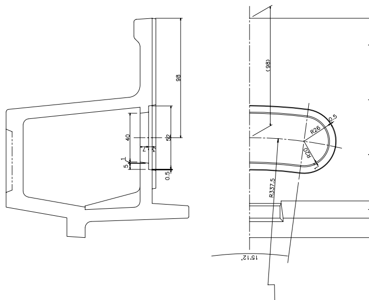
B-B断面图
