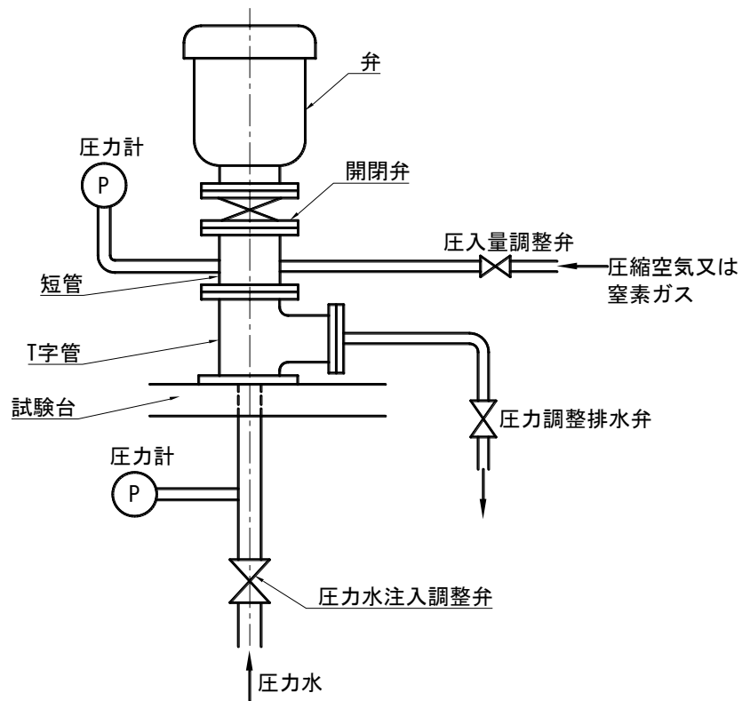
図－１ 試験装置の例
