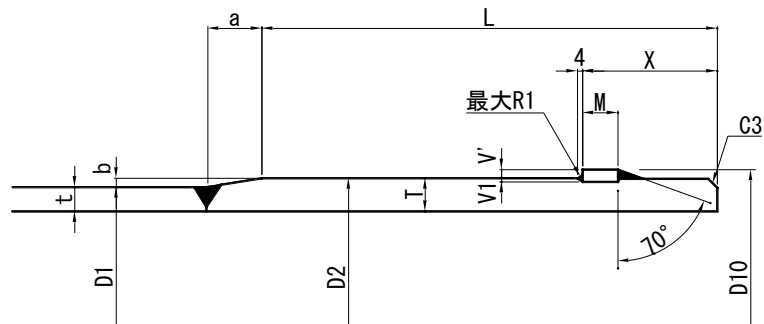
U S 形挿し口寸法図（直管、異形管及び継ぎ輪用）
