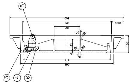
B-B断面图
