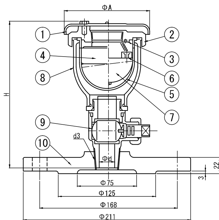
付図－１ 水道用小型急速空気弁
