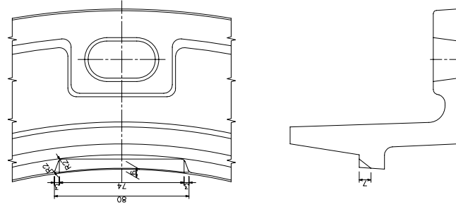
受枠バルブあな部① 詳細図
