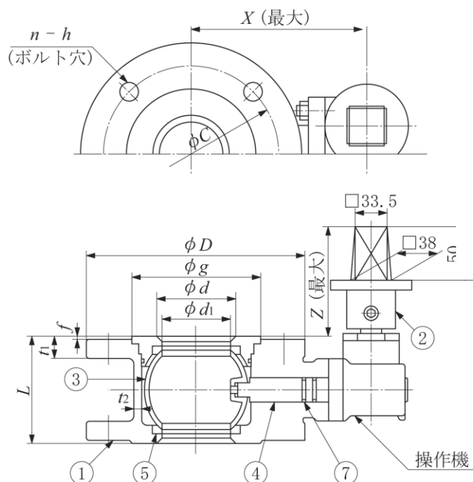
2 種, 呼び径 75, 面間寸法 L = 100 mm の形状
