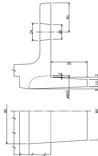
B-B断面図
