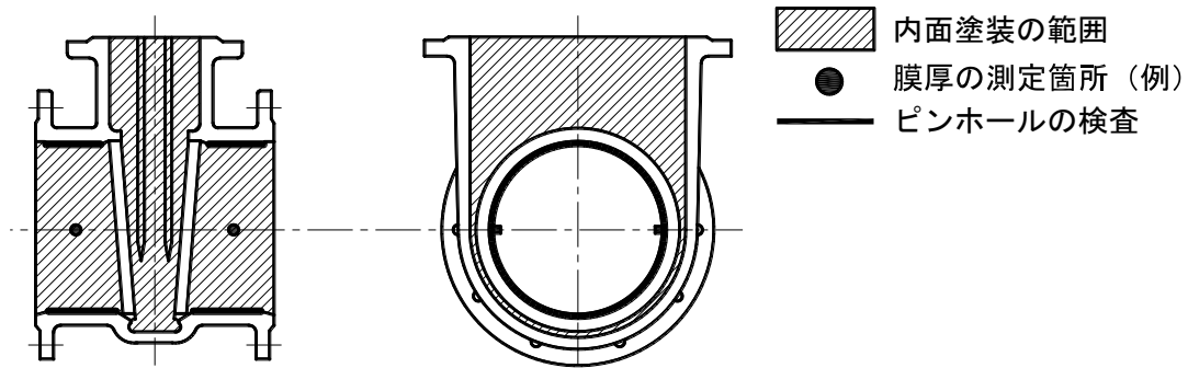
図－１．１ 弁箱の内面塗装範囲及び塗装検査の範囲
