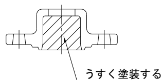
パッキン箱
