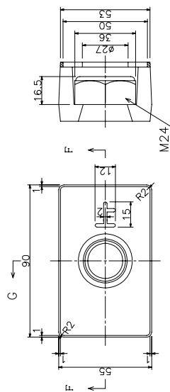
G-G断面图
