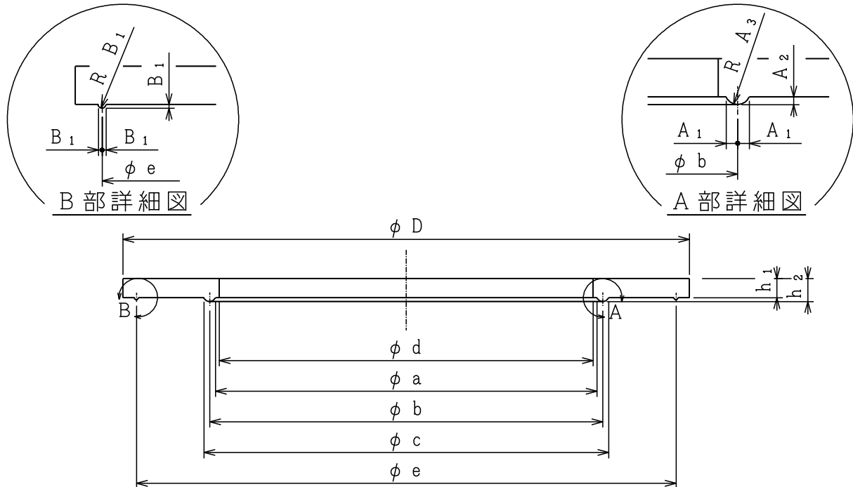
付表－３ 大空気孔弁座寸法
