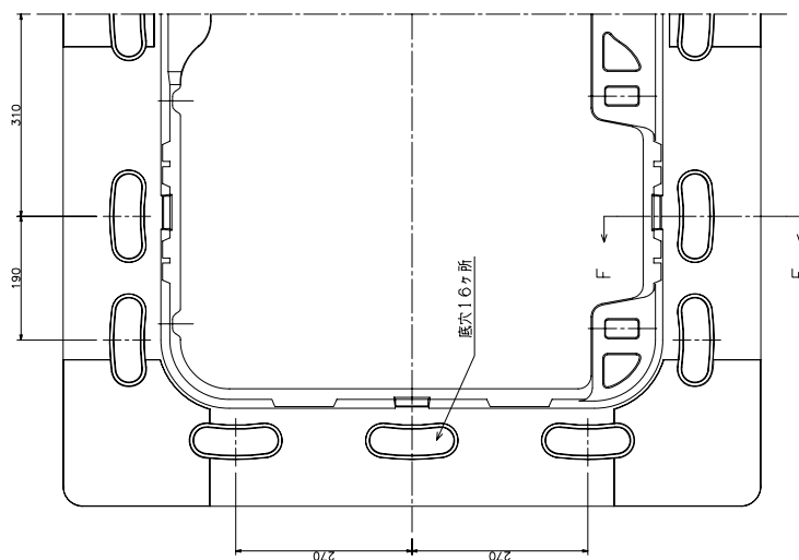
受杵裏面図
