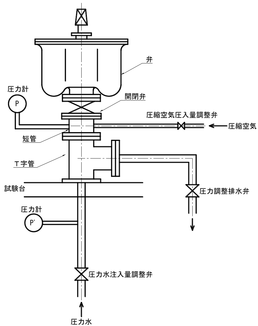
図－１ 試験装置の例
