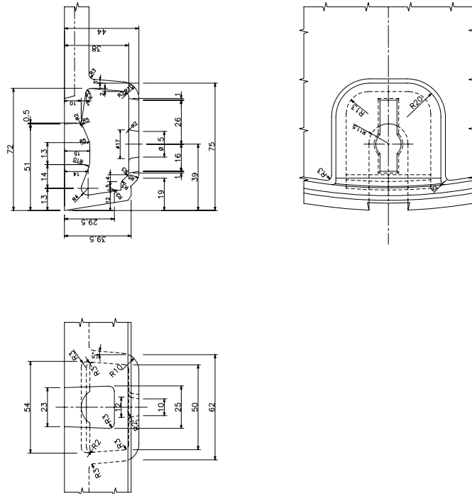
蓋バルブあな部① 詳細図
