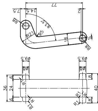
蝶番詳細図
