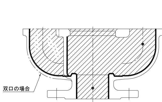
継ぎ足し管
