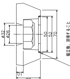
F-1断面图
