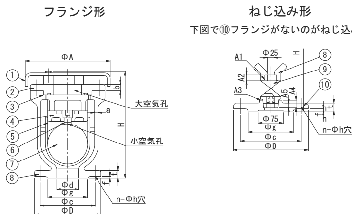
付図－１ 水道用急速空気弁（ねじ込み形 呼び径 13～20）
