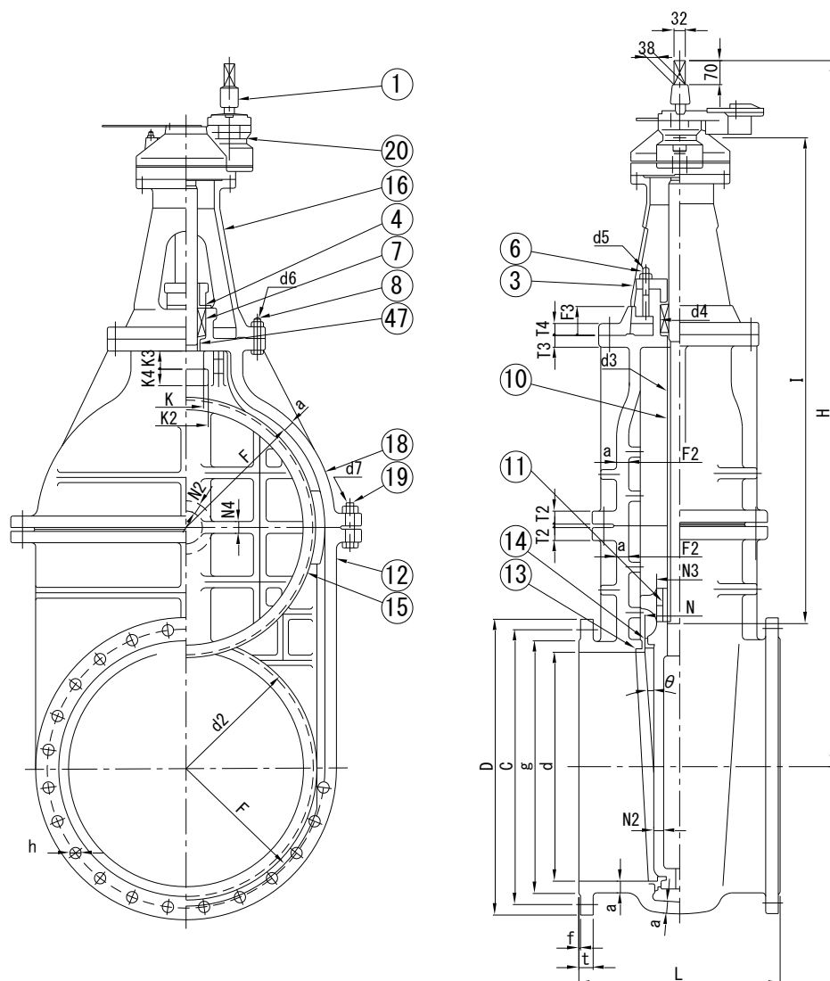
付図-4 水道用ダクタイル鋳鉄仕切弁(呼び径 600~1500:7.5K)立形
