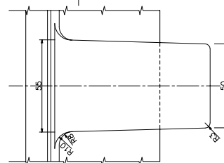
受杵D矢視圖
