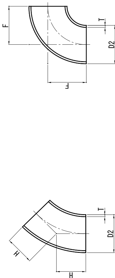
45° エルボ
