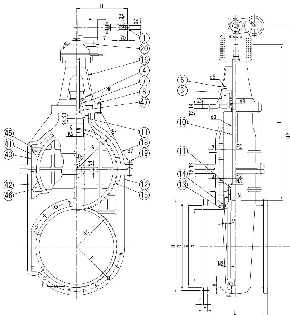
付図－5 水道用ダクタイル鋳鉄仕切弁(呼び径 400～1500:7.5K)横形
