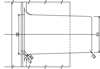
受枠D矢視図
