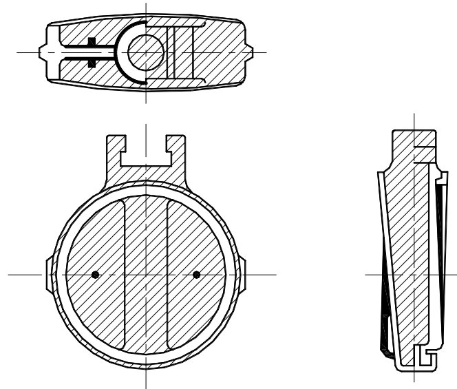
図－１．２ 弁体の内面塗装範囲及び塗装検査の範囲
