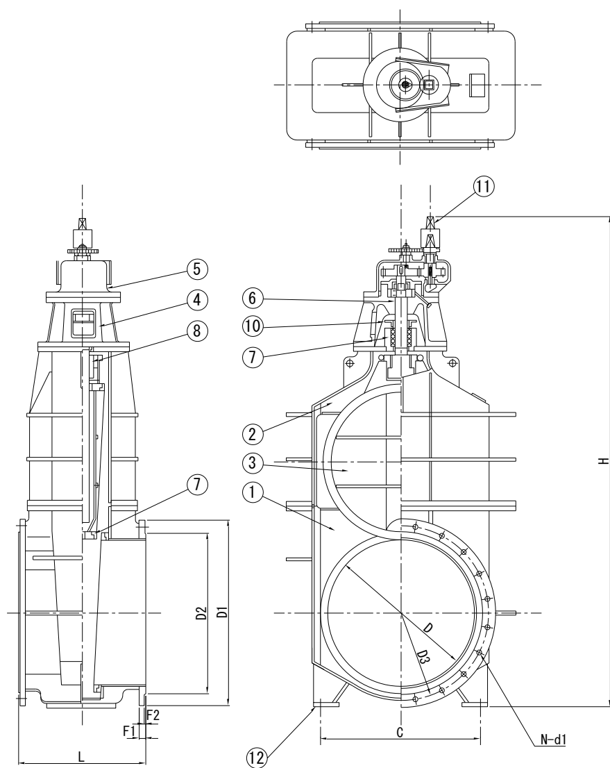
付図－1 水道用鋼板製仕切弁(呼び径 500～2600)立形
