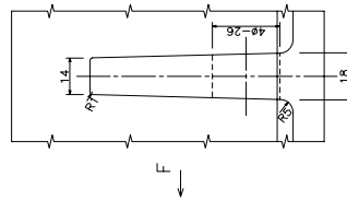
受杵F矢視圖
