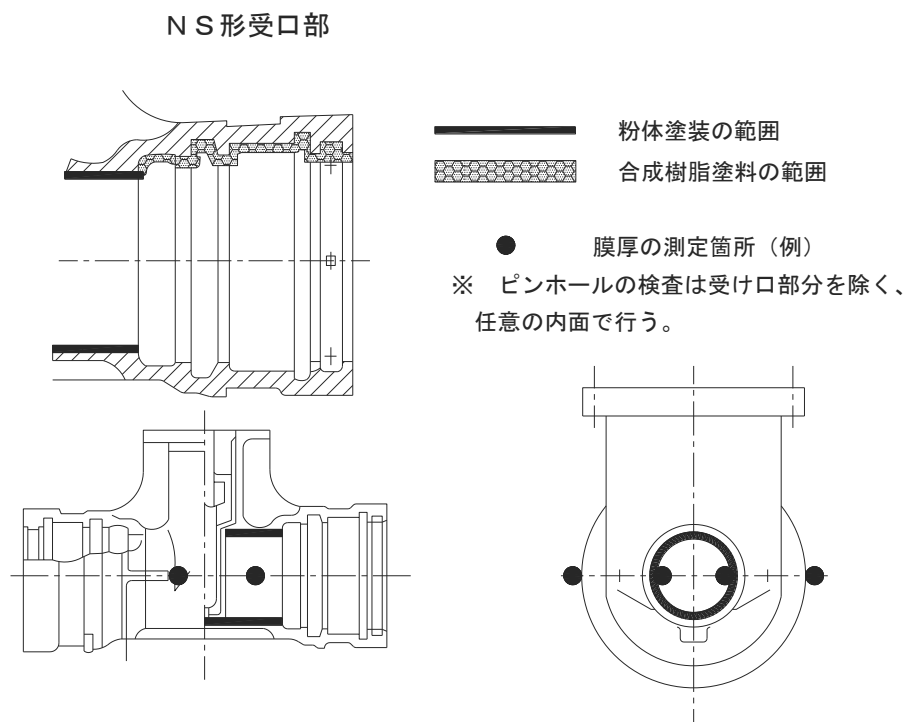
図－3．1 弁箱の内外面塗装範囲、塗装色、塗膜厚及び塗装検査の範囲
