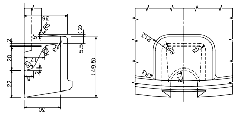
蓋バルブ穴部② 詳細図
