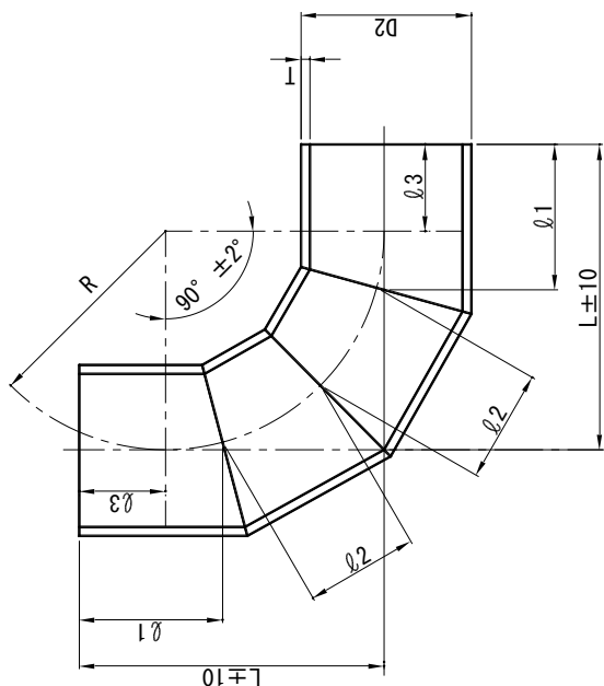
90° 曲管
