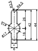
鍵あな詳細図
