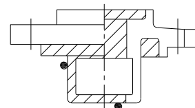
弁箱蓋
