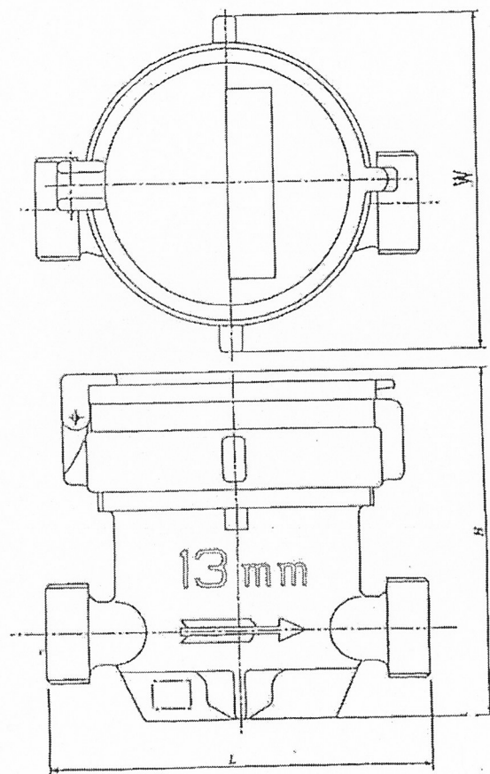
外殻(最大)寸法表 単位 mm
