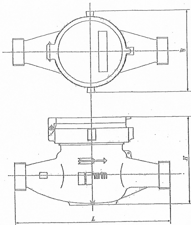
外殻(最大)寸法表
