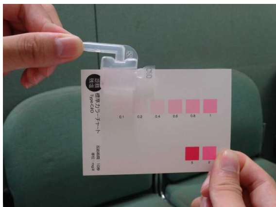
図 31 シンプルパック (遊離残留塩素測定用)
