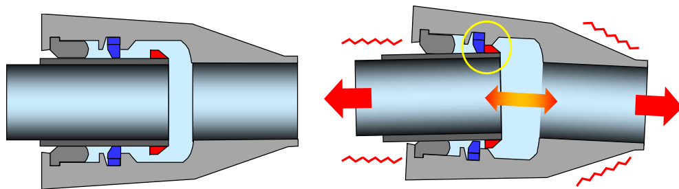
図 8 耐震継手構造…震災時においても継手離脱しない構造 (左図：通常時 右図：震災時)
