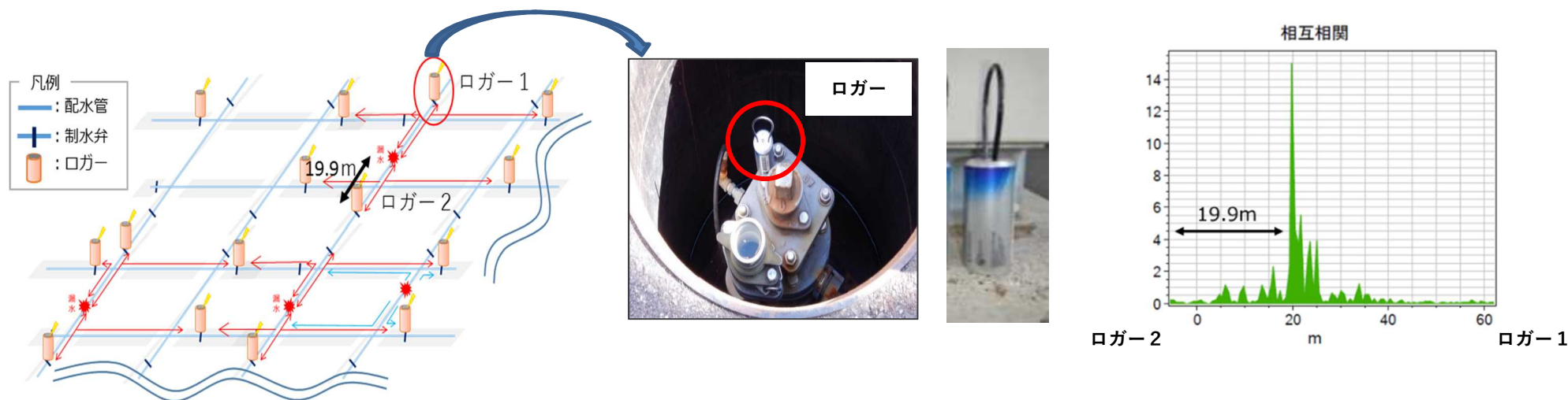
図 28 多点相関式漏水発見器
