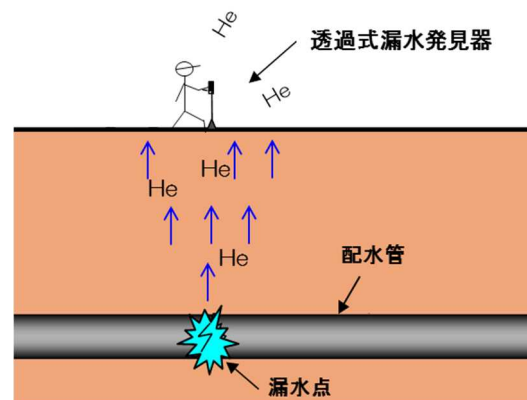
図 27 透過式漏水発見器
