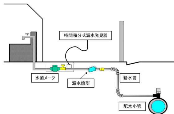
図 26 時間積分式漏水発見器
