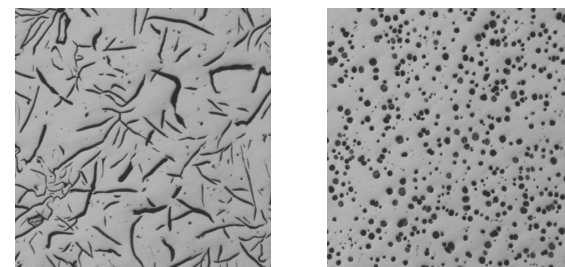
図 9 铸铁の組織 (左図：高級铸铁 右図：ダクタイトイル管)
