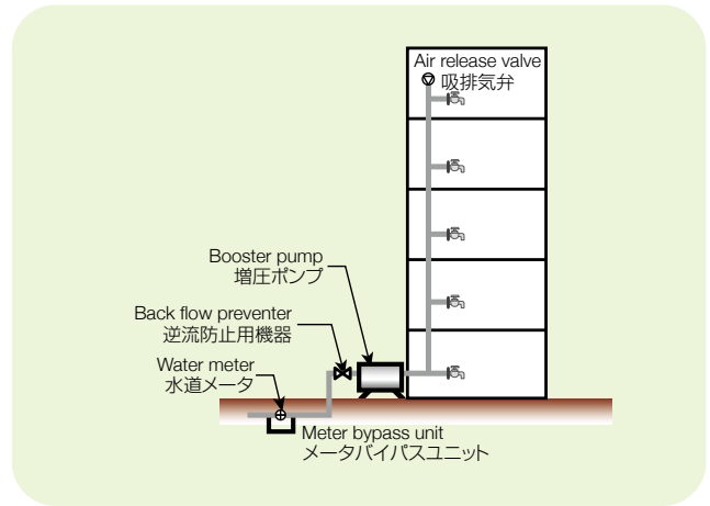
Figure: Pressure Water Service System (standard type) 増圧直結給水方式（標準型）
